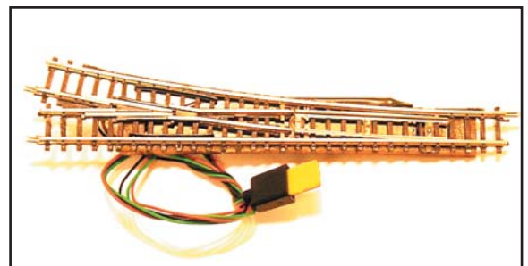
Umgebaute Weiche mit Unterflurantrieb
